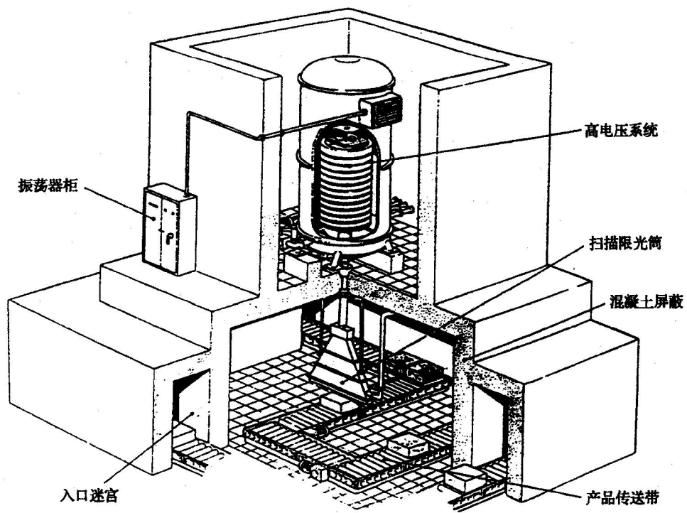
图 A.6 第Ⅱ类电子束辐照装置:安装在屏蔽室内的加速器辐照装置
