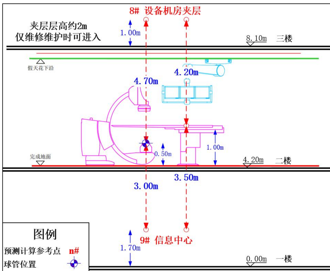
图 11-2 本项目 DSA 机房周围预测点布设纵剖面示意图
