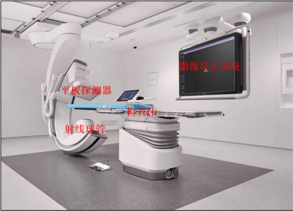
图 9-1 本项目 DSA 外观图
