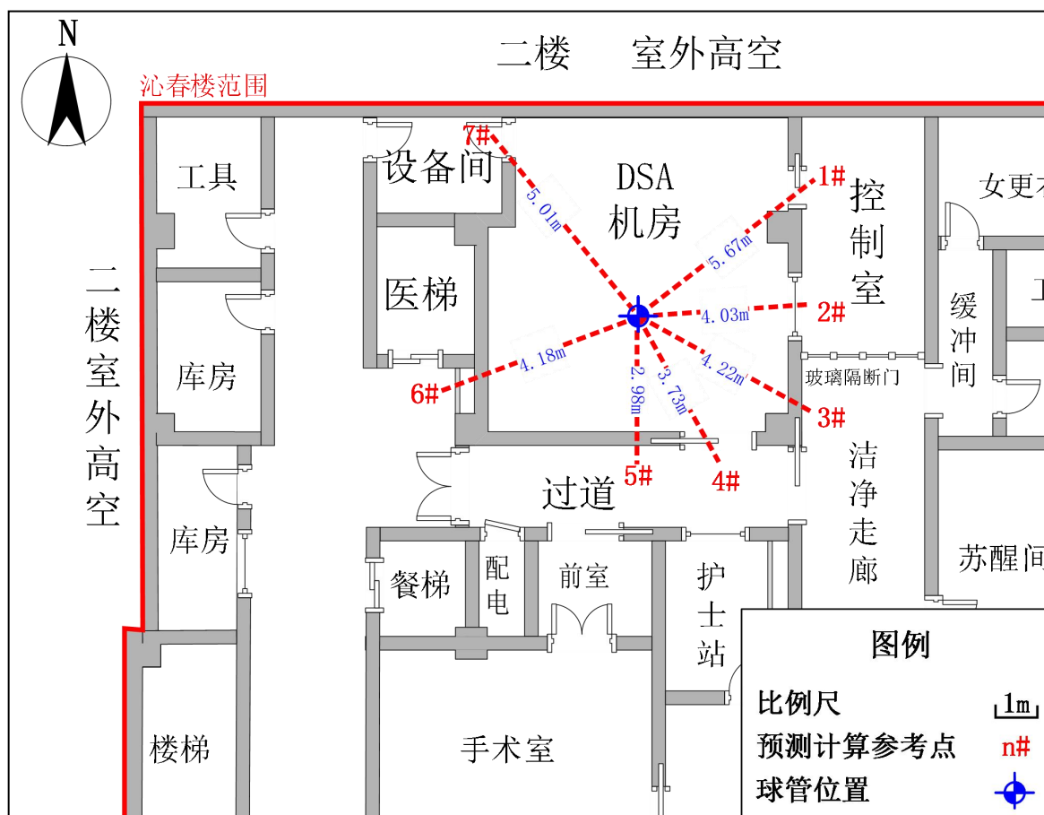
图 11-1 本项目 DSA 机房周围预测点布设平面示意图
